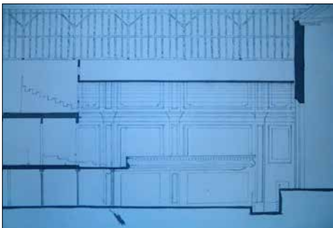
Längsschnitt durch das Theaterschiff
