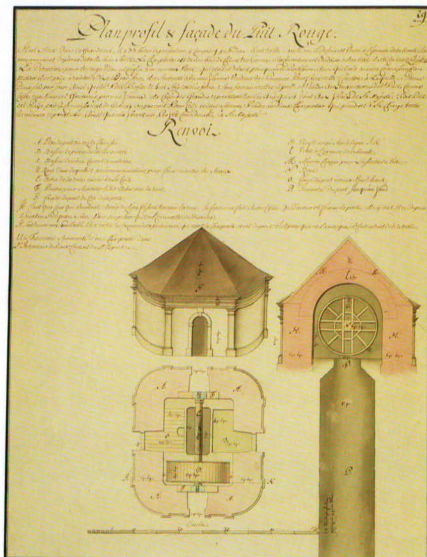
Le Puits Rouge (Atlas des bâtiments militaires)
