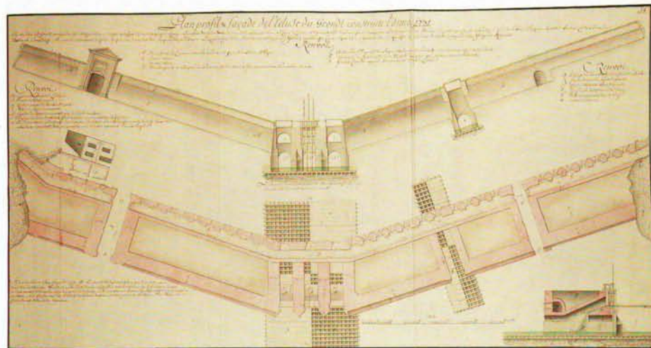
L'écluse du Grund (Atlas des bâtiments militaires)
